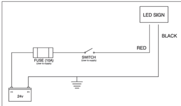
Wiring Guide
